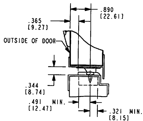
060-0201内旋门无内置锁舌锌压铸冲击板
