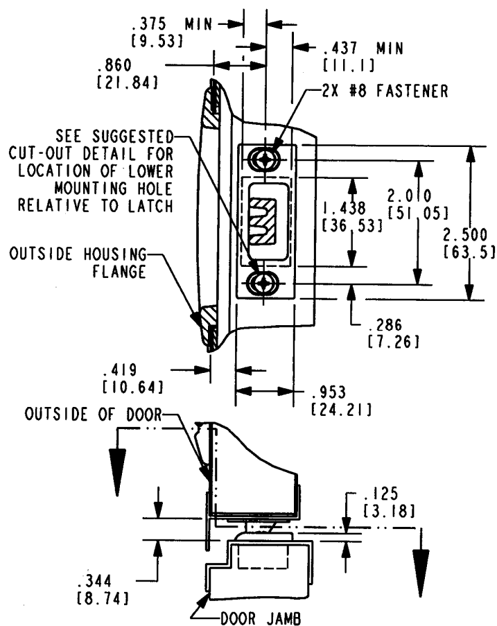
060-0201无内置锁舌锌压铸冲击板
